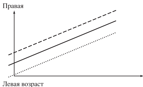
Рис. 1. Роль коэффициента \beta_2 (схематично).
