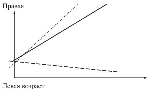
Рис. 2. Роль коэффициента \beta_3 (схематично).
